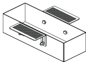
Cassaforma CA155
